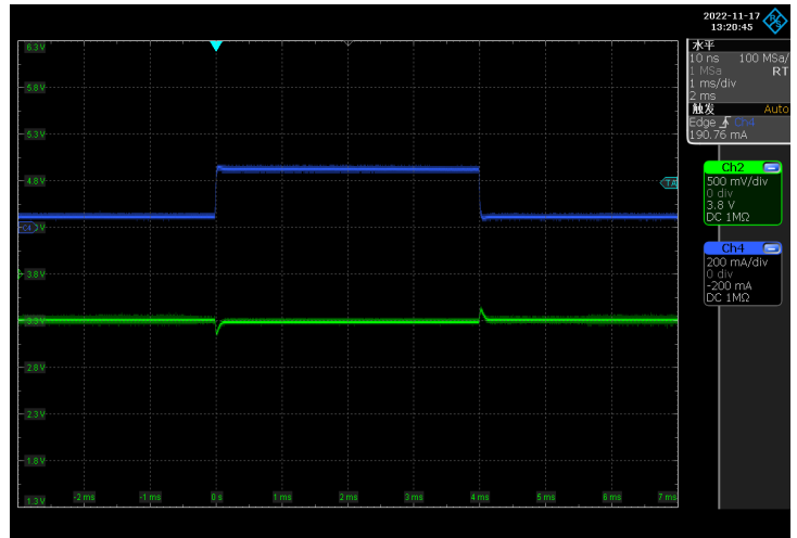
I_{OUT}: 50 \sim 250\text{mA}
