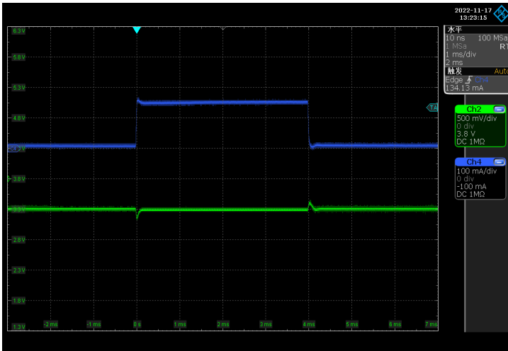
I_{OUT}: 10 \sim 150\text{mA}
