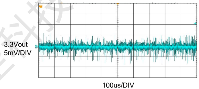
3.3V 输出纹波-4A负载
