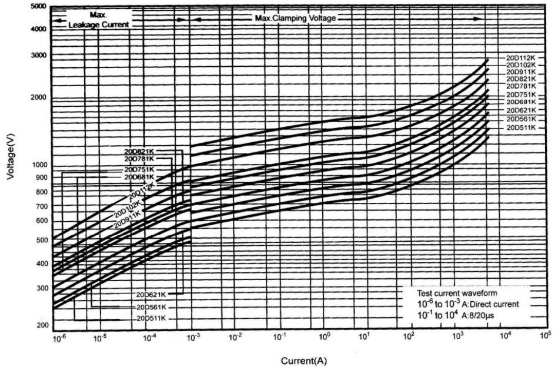
V-I Curve 20D511K to 20D112K 电压-电流特性曲线
