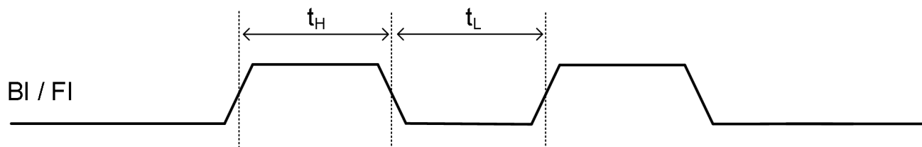
图 5. 输出时序图
