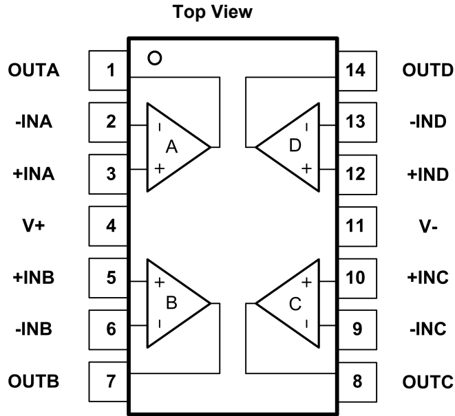
Fig.5-4. GT8554: PD(SOIC-14/SOP14) Package GT8554: TD(TSSOP14) Package
