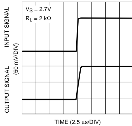
图 22. 小信号同相响应
