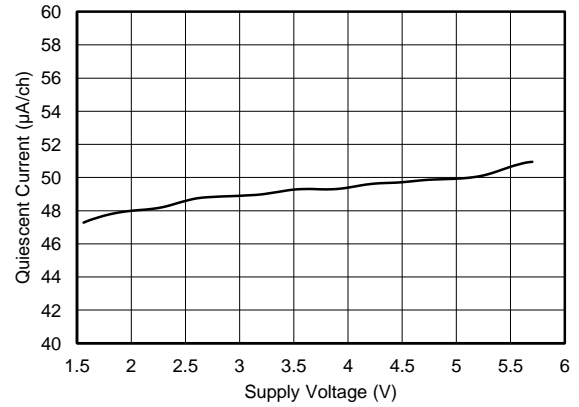
图 2. 静态电流与电源电压间的关系
