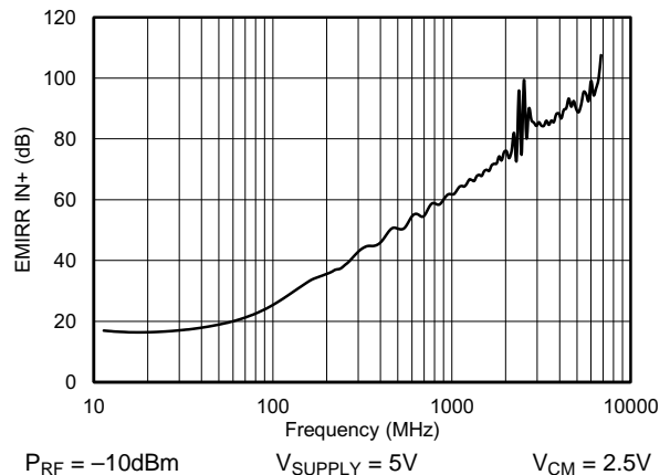
图 18. EMIRR IN+ 与频率间的关系
