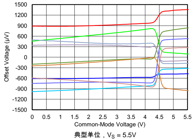
图 4. 失调电压与共模电压间的关系
