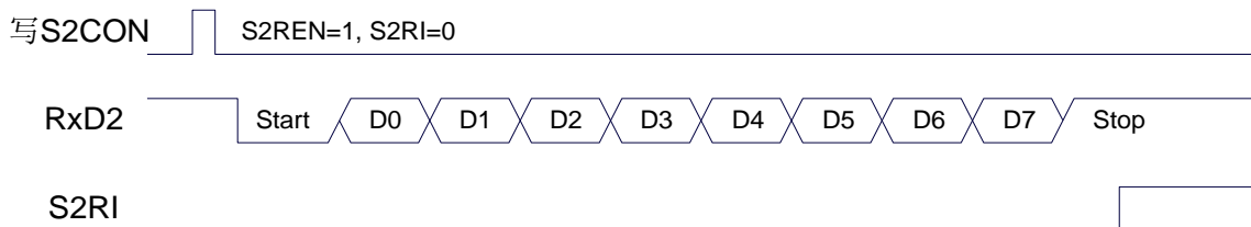
接收数据 (串口2模式1)
