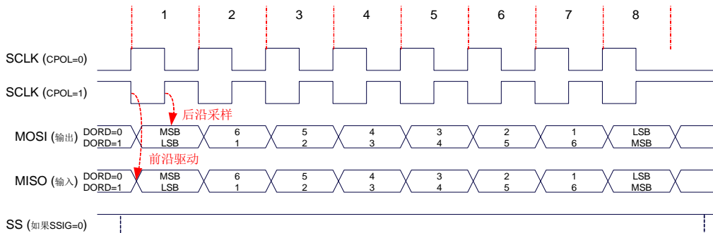
主机传输 (CPHA=1)
