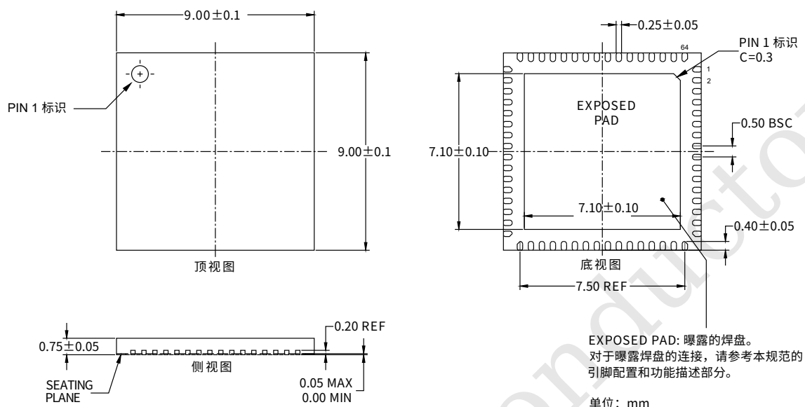
图 15: 封装信息
