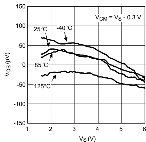
图 6. 输入失调电压与电源电压间的关系
