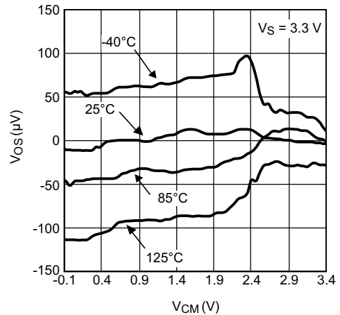
图 4. 输入失调电压与输入共模电压间的关系
