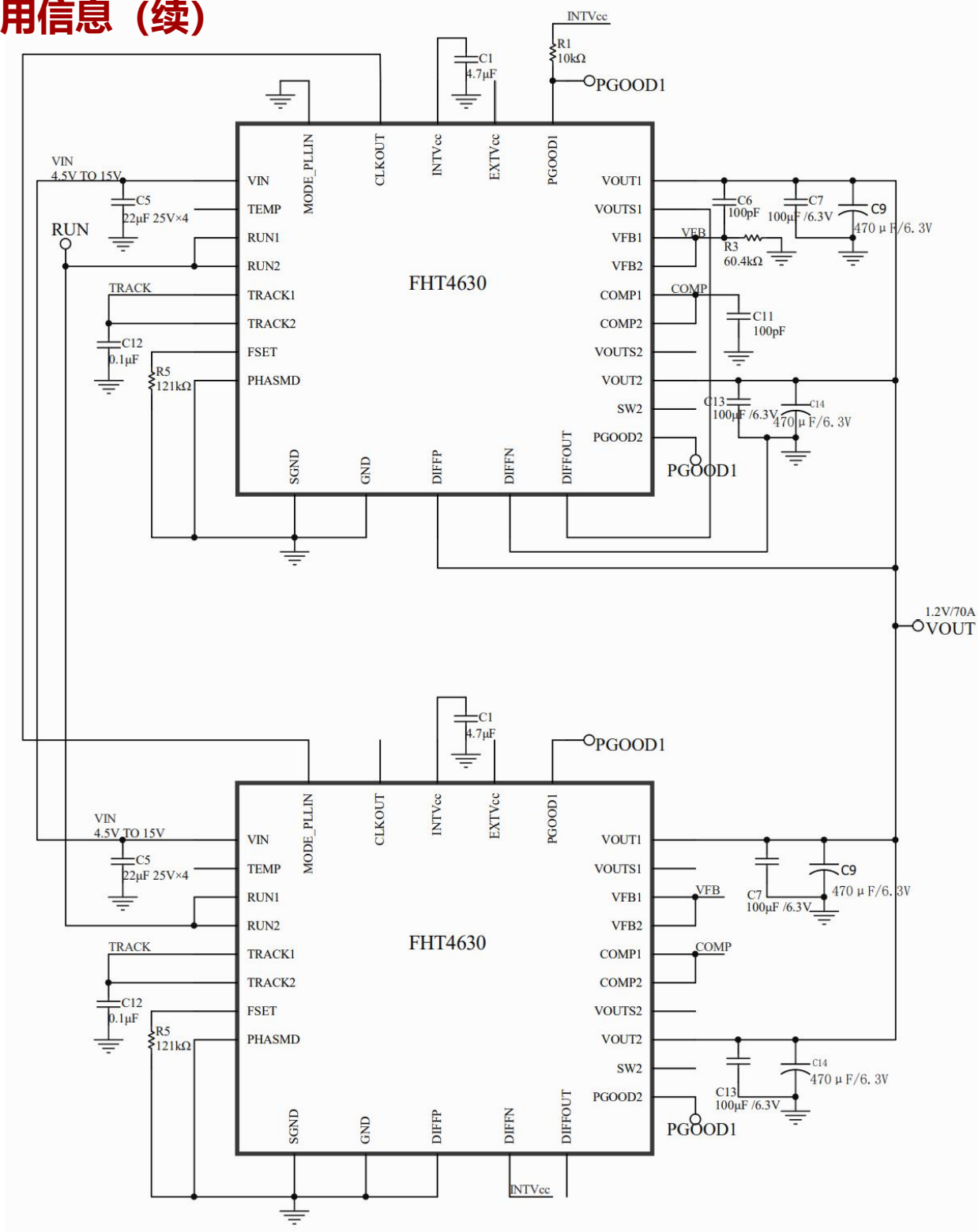
典型电路 4相并联输出应用示例
