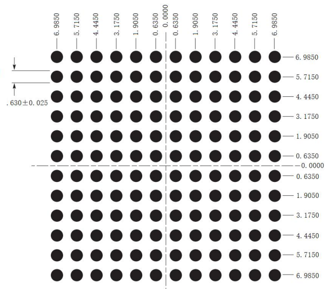
建议焊盘设计
