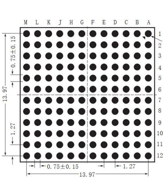
底视图
