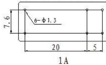
安装脚位图(底视图)
