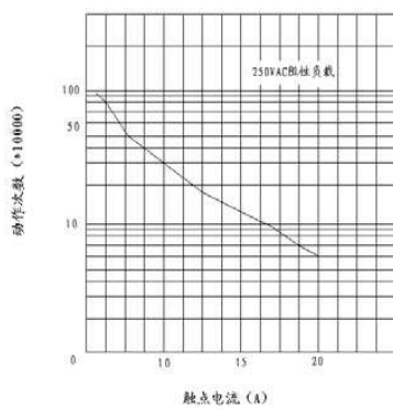
寿命曲线
