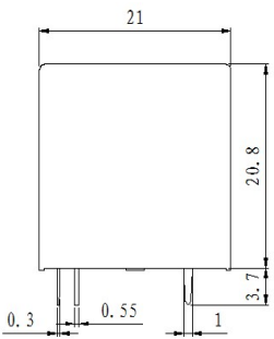
一组常开
