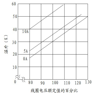
线圈温升
