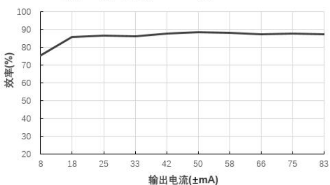
效率Vs输出电流(Vin=12V)@E1212S-2WR3
