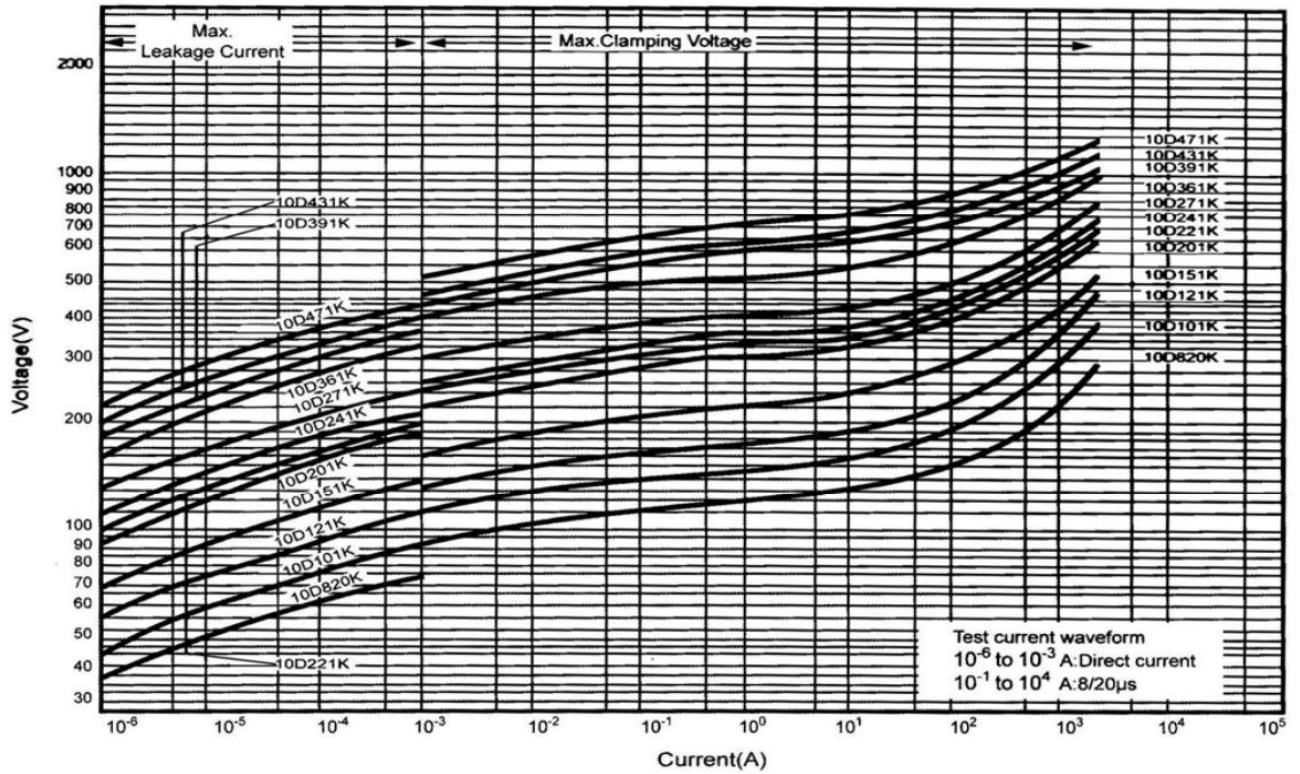
V-I Curve 10D820K to 10D471K 电压-电流特性曲线
