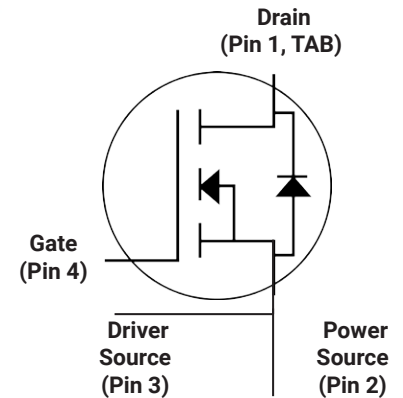
TO-247-4
