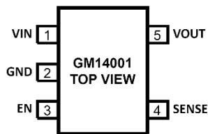
图 4.5 引脚 SOT 引脚配置
