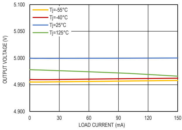
图 12. 5.0V 输出电压和负载电流的关系
