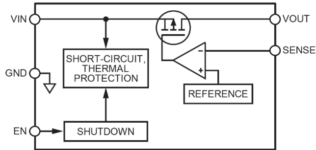
图 24. 内部框图
