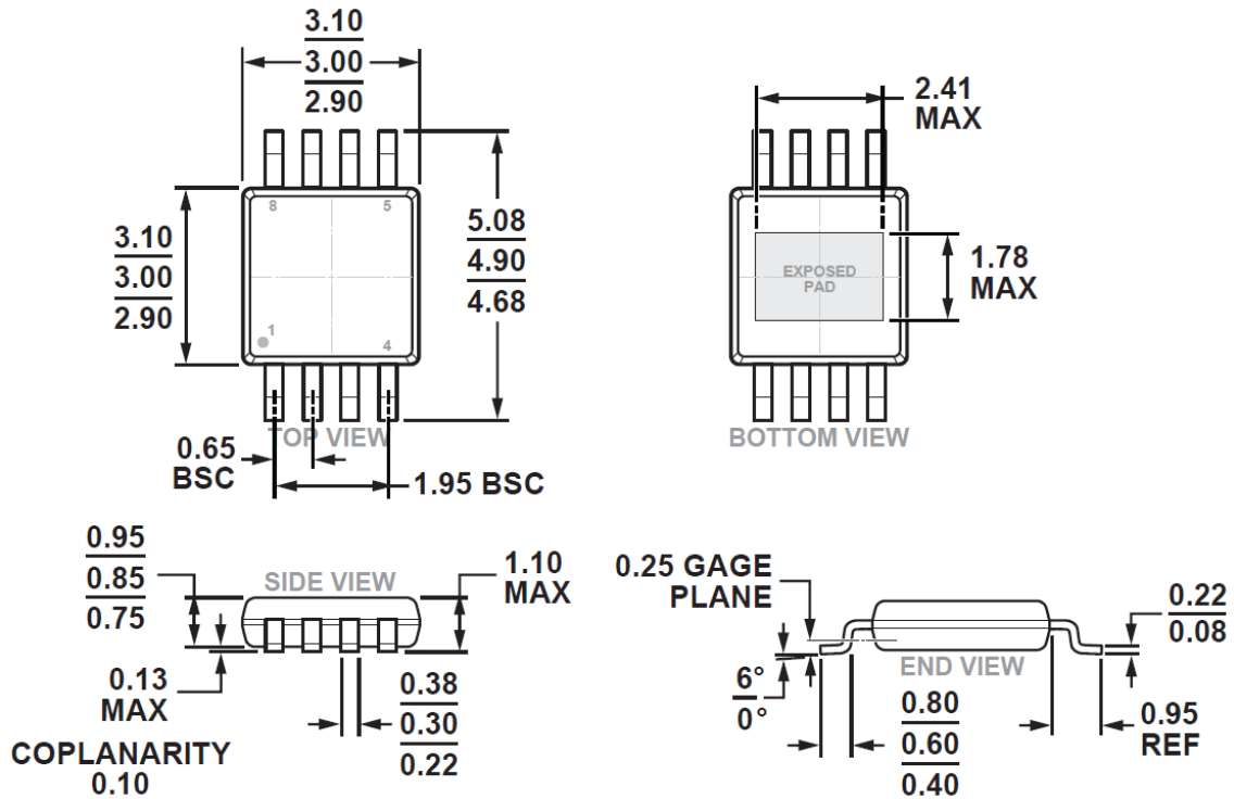
图 32.8 引脚 MSOP
