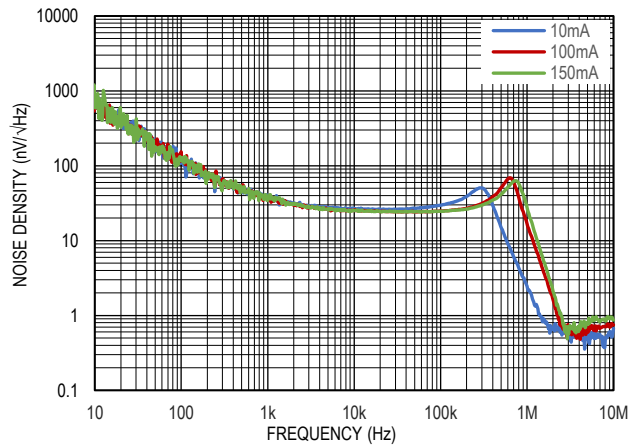
图 17. 输出噪声谱密度, V_{\text{IN}}=5\text{V} , V_{\text{OUT}}=3.3\text{V}
