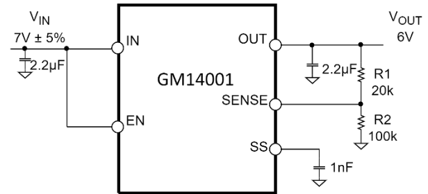
图 25. 典型可调输出电压应用原理图
