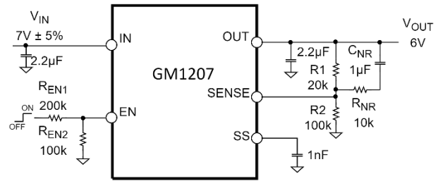
图 28. 噪声优化
