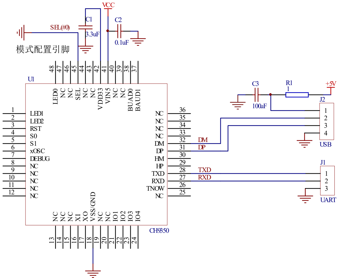
图 7-2 上位机模式
