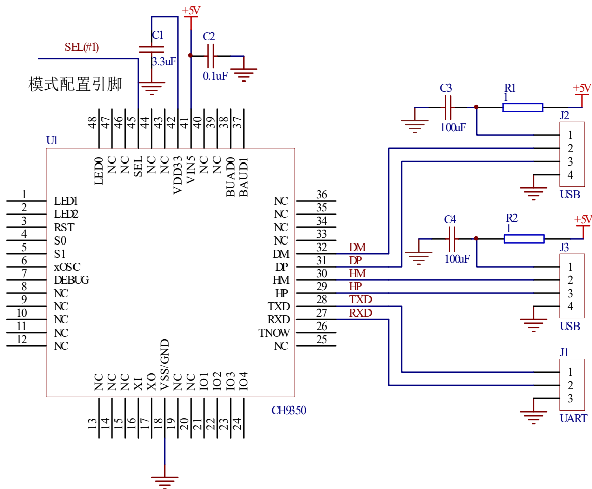
图 7-1 下位机模式
