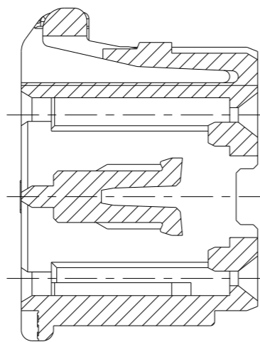
A - A
