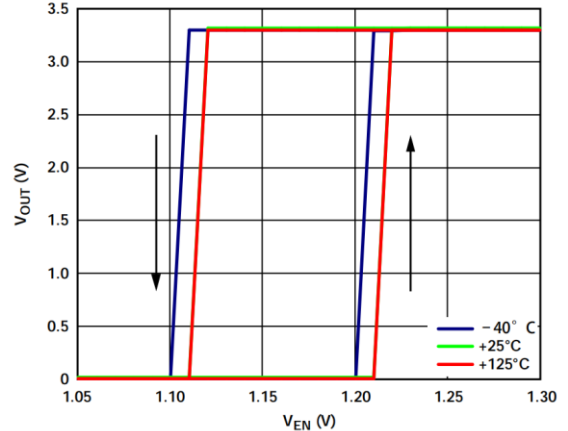
图 29. 对 EN 引脚工作方式的典型 V_{OUT} 响应
