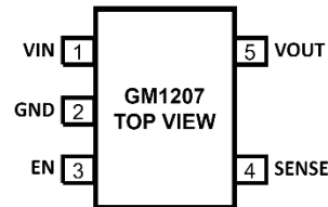
图 4.3 引脚 SOT-23 引脚配置
