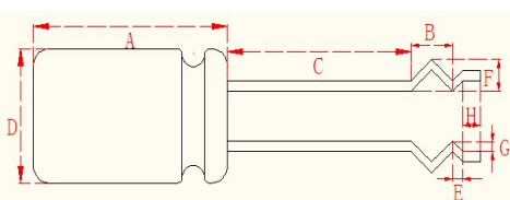
引线切脚成型 C 图
