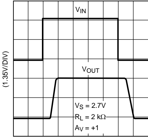
TIME (10 \mu s /DIV) 图 25. 大信号同相响应
