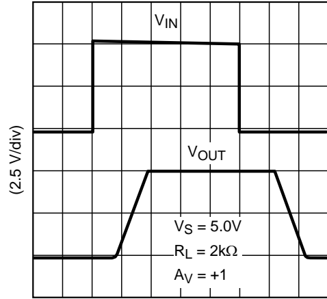
TIME (10 \mu s /div) 图 26. 大信号同相响应
