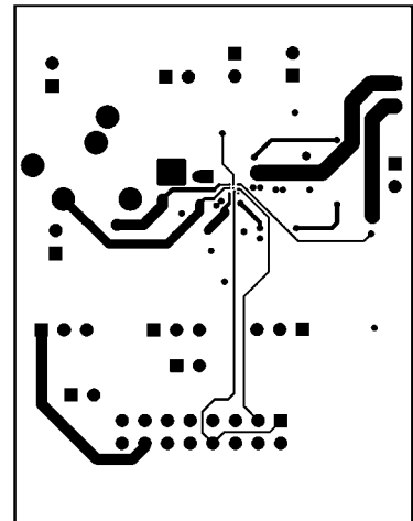
Bottom Layer
