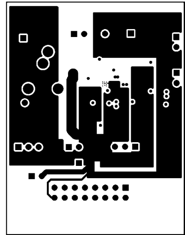
Internal Layer 1
