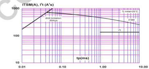
6、 I_{TSM}-t, I^2t-t 曲线
