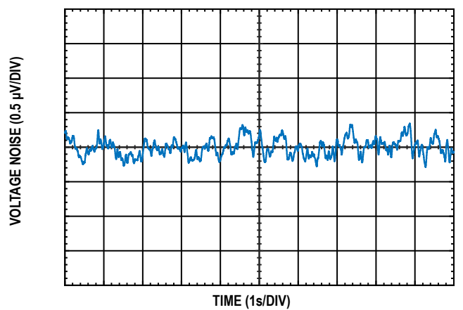
图23. 0.1 Hz 至 10 Hz RTI 电压噪声 ( G = 100 )
