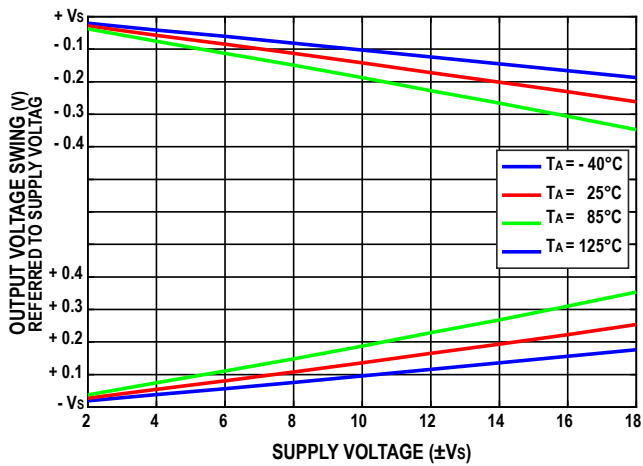
图20. 输出电压摆幅与电源电压的关系 ( G = 1, R_L = 2\text{ k}\Omega )
