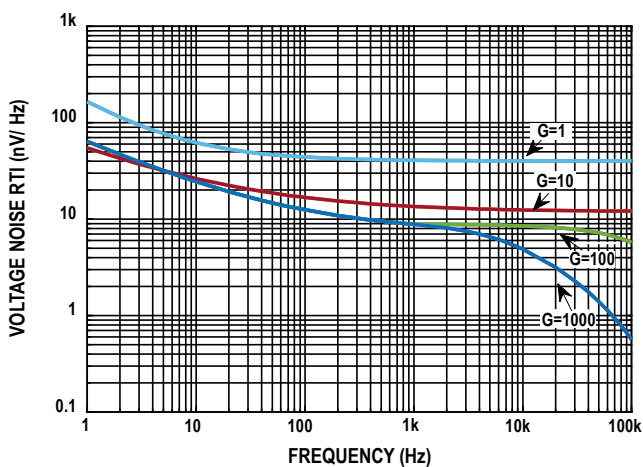
图24. 电压噪声谱密度与频率的关系 ( G = 1 至 1000)
