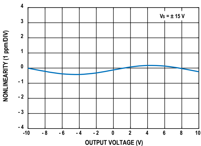
图22. 增益非线性度 ( G = 1, R_L = 10\text{ k}\Omega )
