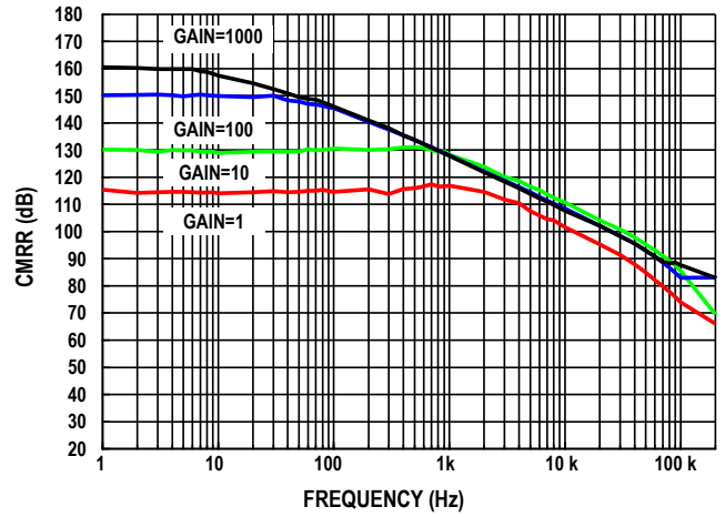
图15. CMRR与频率的关系 (RTI)
