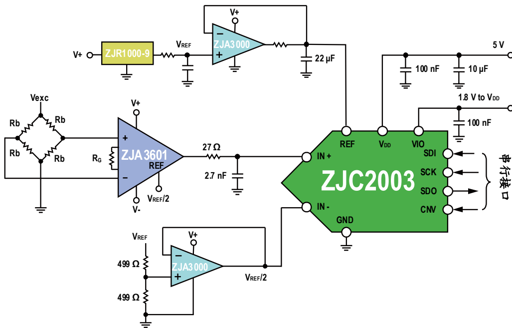
图35. 桥式电路与 ZJA3601 接口
