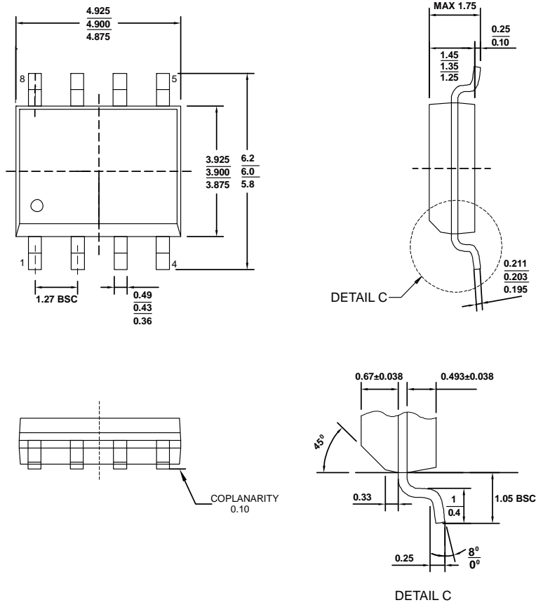
图41. SOIC-8 封装尺寸图 (单位: 毫米)
