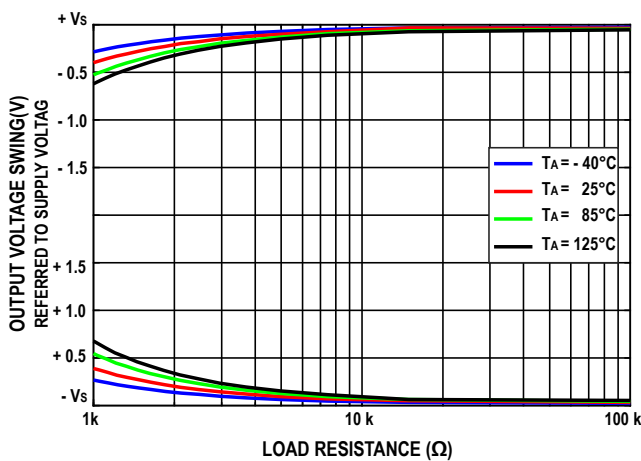
图18. 输出电压摆幅与负载电阻的关系
