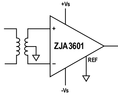
图32. ZJA3601 与变压器的连接
