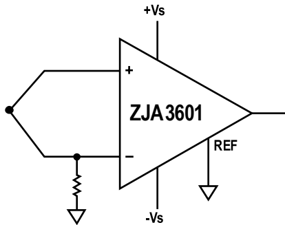
图31. ZJA3601 与热电偶的连接
