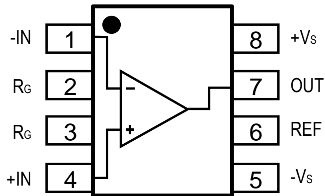
图1. ZJA3601 管脚排列图
