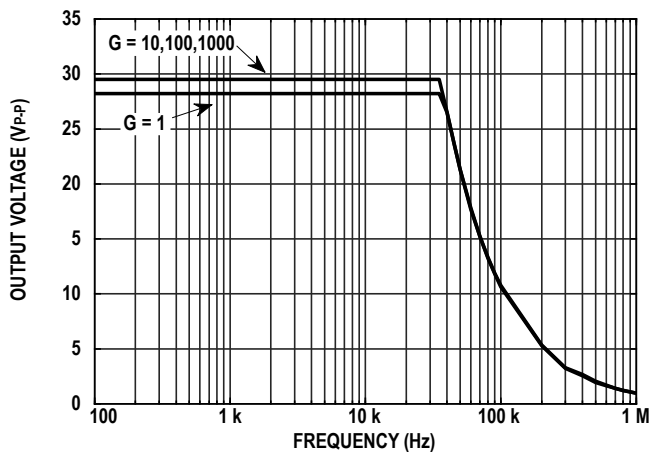
图25. 大信号频率响应
