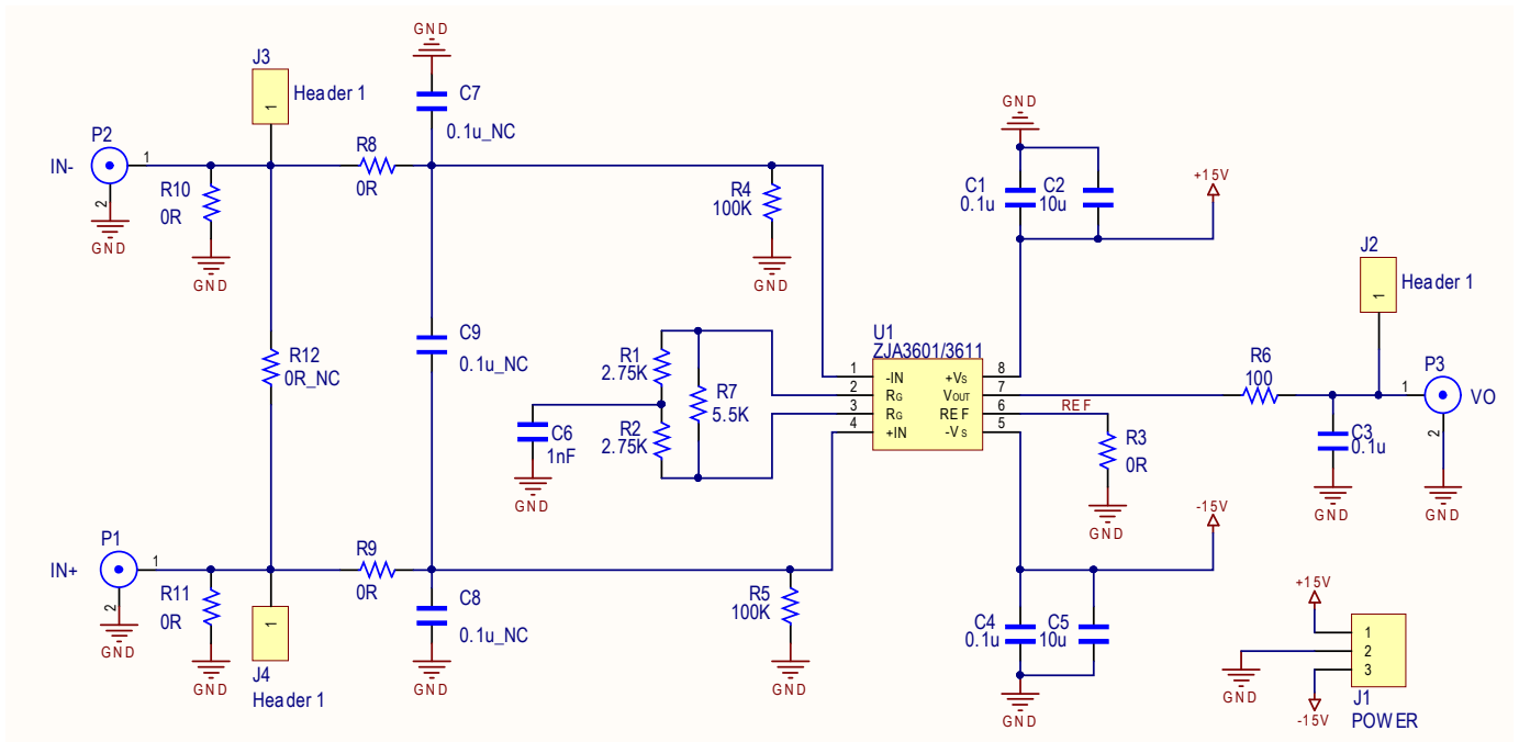
图 38. ZJA3601/3611 评估板原理图
