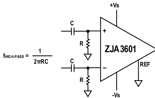
图33. ZJA3601 的交流耦合接法
