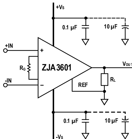
图34. ZJA3601 电源去耦示意图
