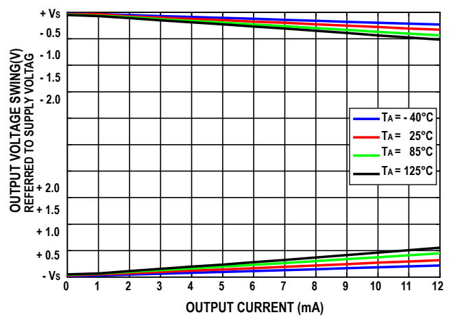
图21. 输出电压摆幅与输出电流的关系 ( G = 1 )
