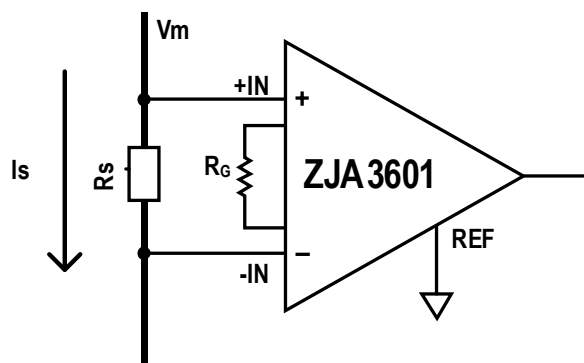
图37. ZJA3601 用于精密电流检测
