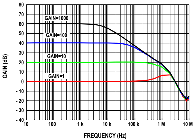
图14. 增益与频率的关系
