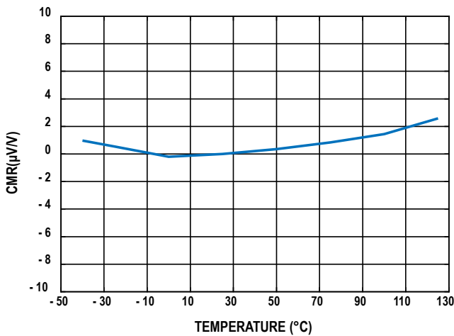
图16. CMR与温度的关系
