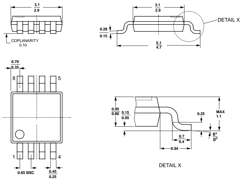
图42. MSOP-8 封装尺寸图 (单位: 毫米)
