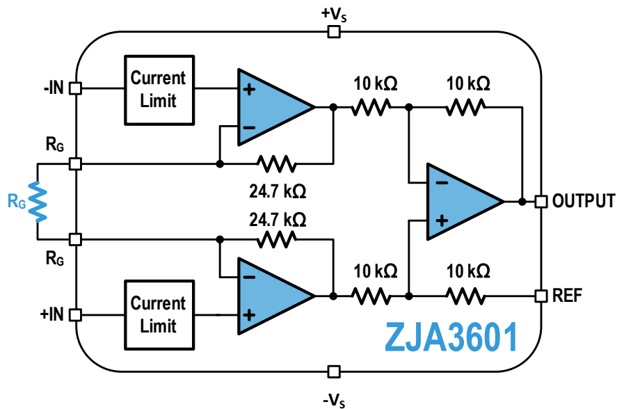
图30. ZJA3601 简化的示意图
