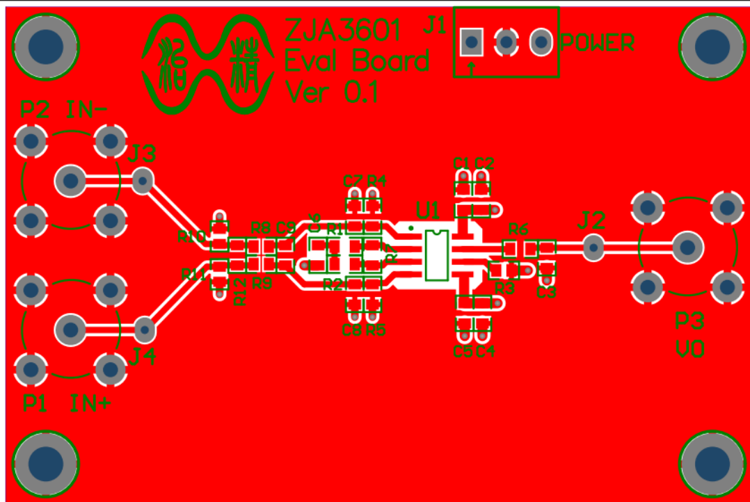
图39. ZJA3601/3611 评估板 PCB 顶层设计
