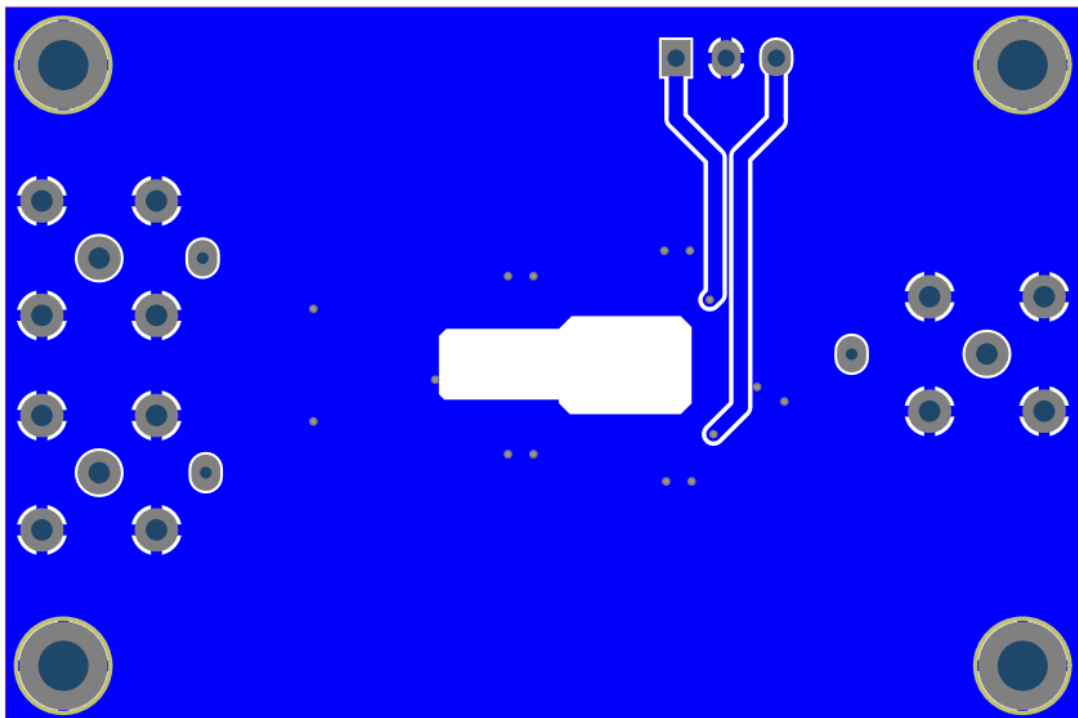
图40. ZJA3601/3611 评估板 PCB 底层设计
