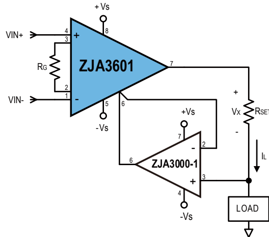
图36. 用 ZJA3601 构建精密电流源
