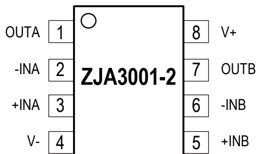
ZJA3001-2引脚配置 SOIC-8封装和MSOP-8封装
