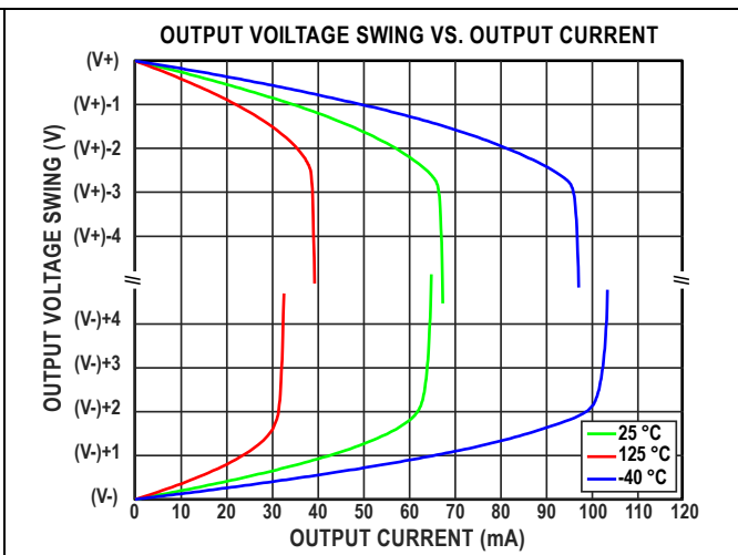
图32. 输出电压摆幅与输出电流的关系
