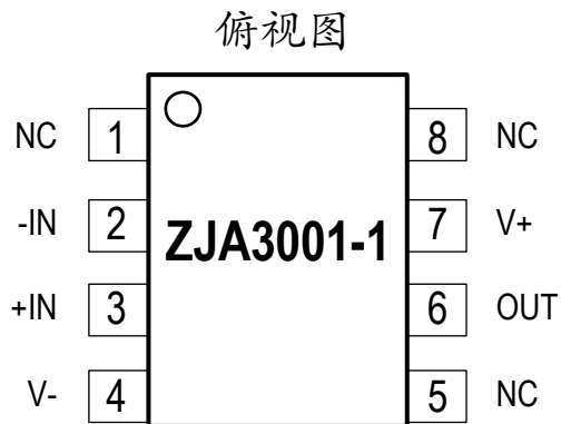
ZJA3001-1引脚配置 SOIC-8封装和MSOP-8封装
