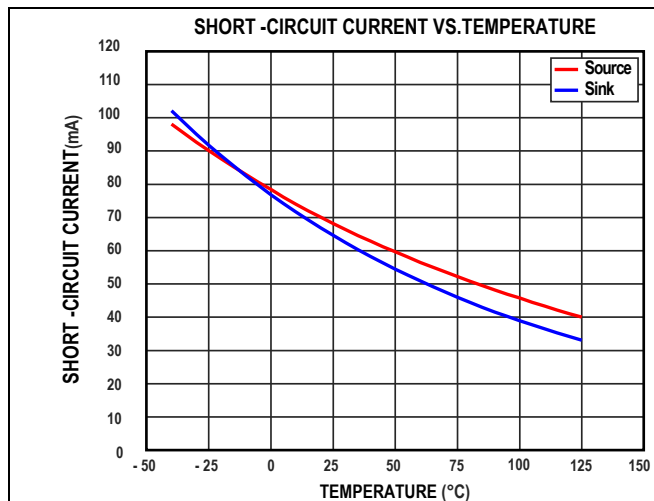
图31. 短路电流与温度的关系
