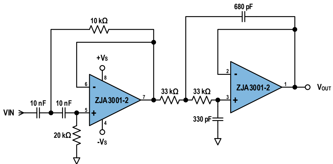
图38. 使用 ZJA3001-2 实现 2 级带通 KRC 滤波器
