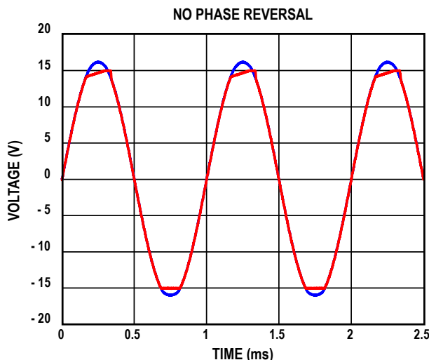
图35. ZJA3001 没有输出相位反转的现象
