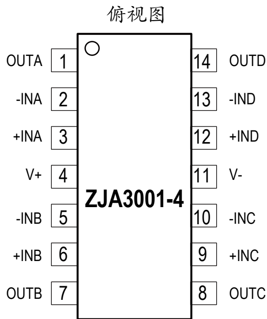
ZJA3001-4引脚配置 SOIC-14封装和TSSOP-14封装
