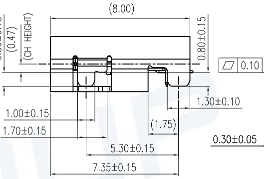
SECT A-A (2:1)
