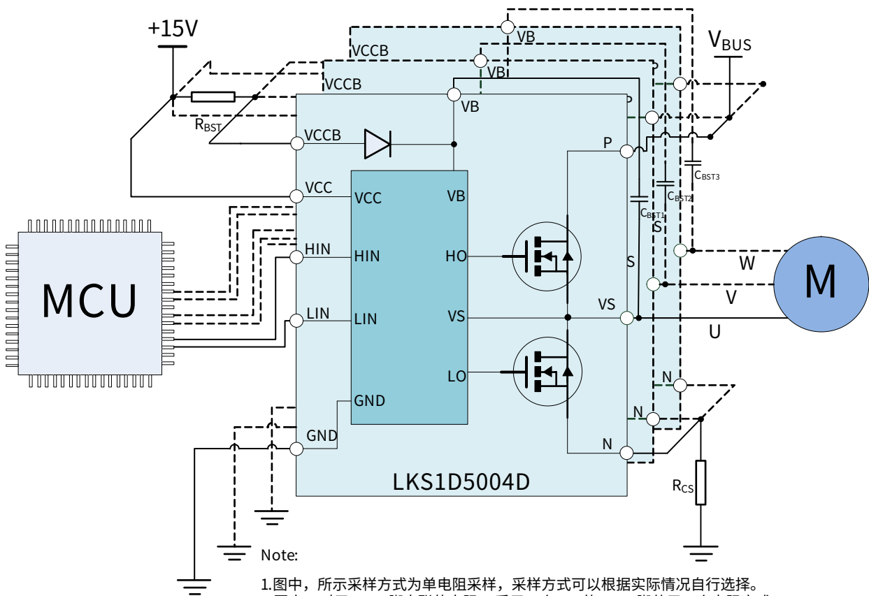
图 1. LKS1D5004D 典型应用图
