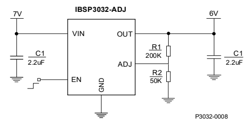
图6.3 IBSP3032输出电压可调的典型应用
