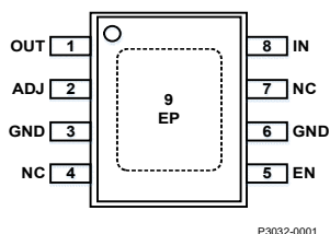
图4.1 SOIC8封装 (4.9mm×6mm×1.4mm)
