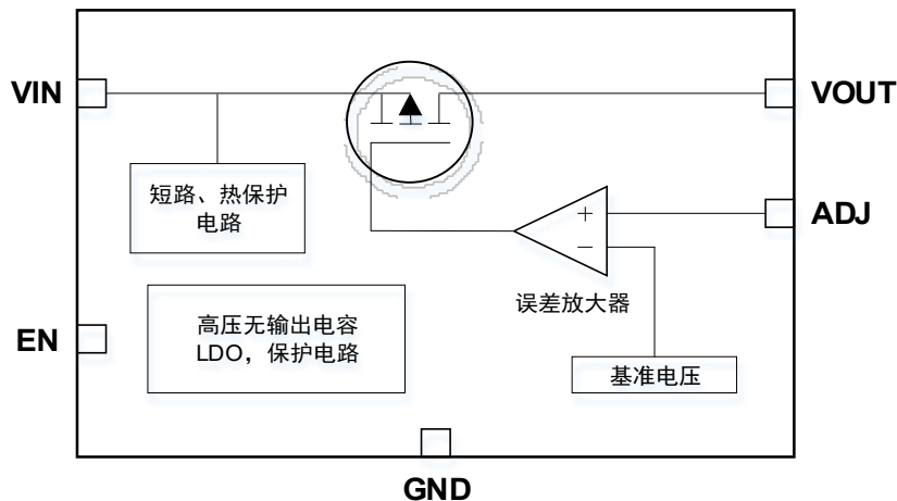
图6.1 IBSP3032功能框图
