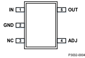
图4.4 SOT23-5 ② 封装 (2.92mm×2.8mm×1.1mm)
