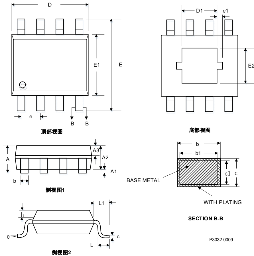
图12.1 IBSP3032 SOIC8封装尺寸
