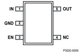
图4.5 SOT23-5 ③ 封装 (2.92mm×2.8mm×1.1mm)
