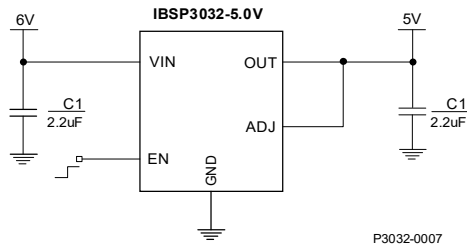
图6.2 IBSP3032输出电压固定的典型应用
