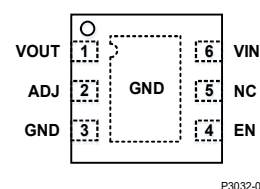
图4.2 DFN6封装 (2mm×2mm×0.73mm)
