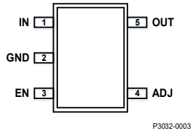
图4.3 SOT23-5 ① 封装 (2.92mm×2.8mm×1.1mm)
