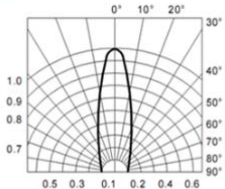
发光角度图解
