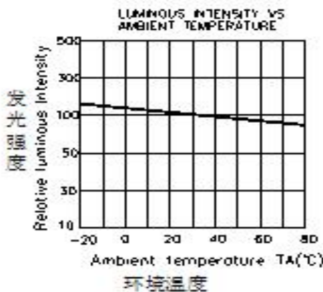
发光强度与环境温度关系
