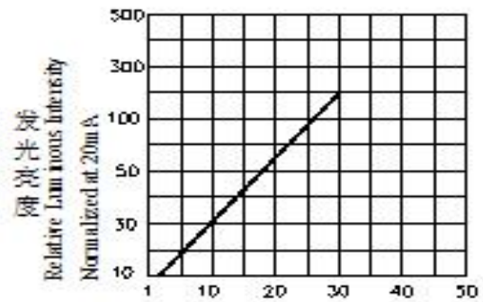
正向电流与发光强度关系 Fig.4 Relative Luminous Intensity vs Forward Current
