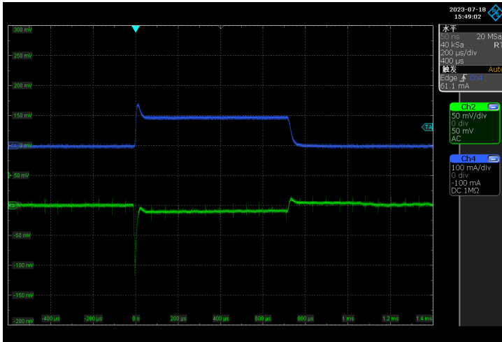
I_{OUT}: 0 \sim 100\text{mA}
