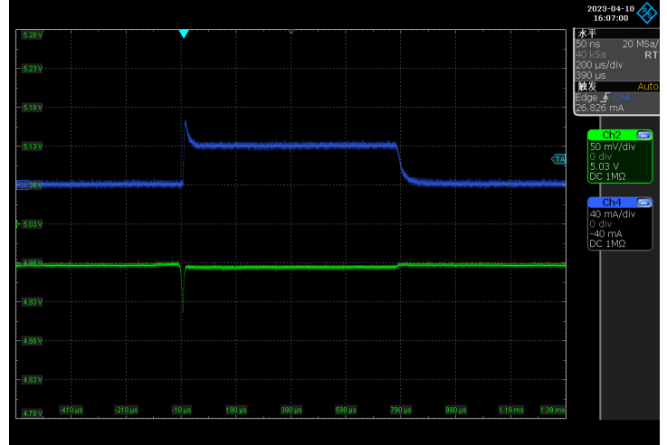
I_{OUT}: 10 \sim 80\text{mA}
