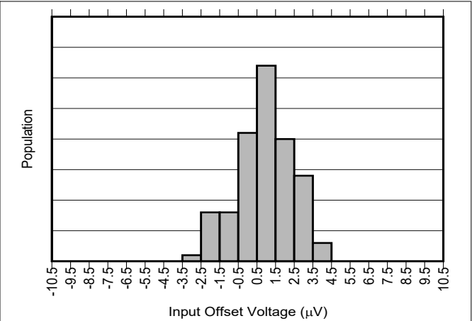
图 7-2. INA241A2-Q1 输入失调电压产生分布图
