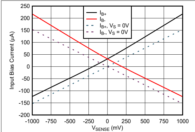
图 7-19. INA241x2-Q1 输入偏置电流与 V_{\text{SENSE}} 间的关系
