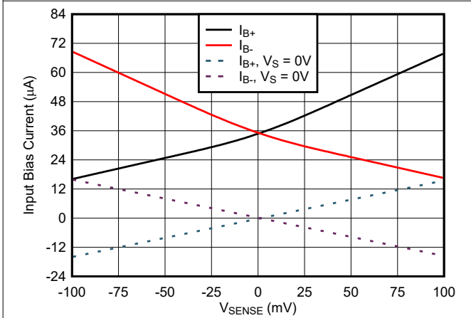
图 7-21. INA241x5-Q1 输入偏置电流与 V_{\text{SENSE}} 间的关系
