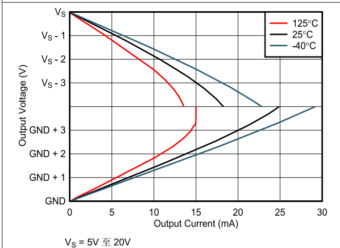
图 7-23. 输出电压与输出电流间的关系
