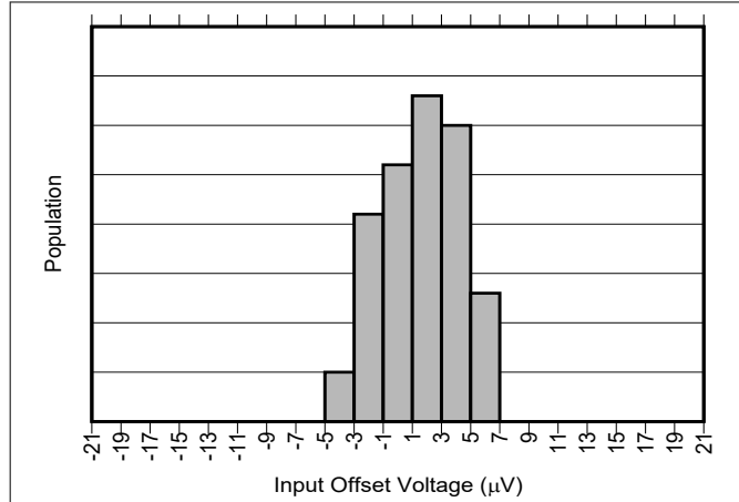
图 7-1. INA241A1-Q1 输入失调电压产生分布图
