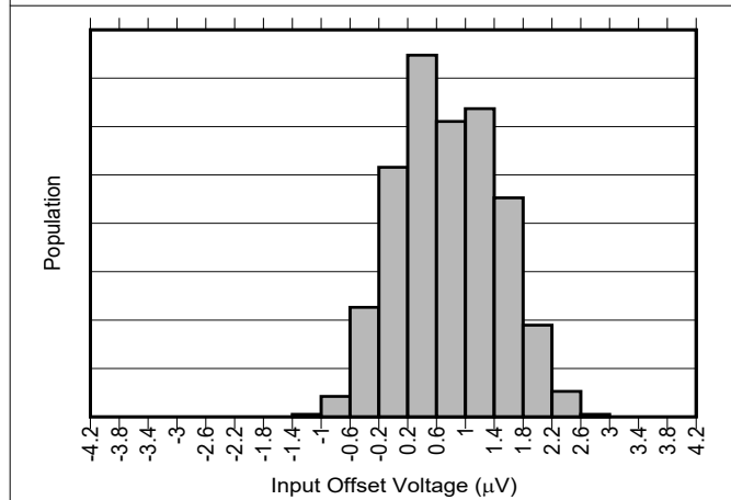
图 7-3. INA241A3-Q1 和 INA241A4-Q1 输入失调电压产生分布图
