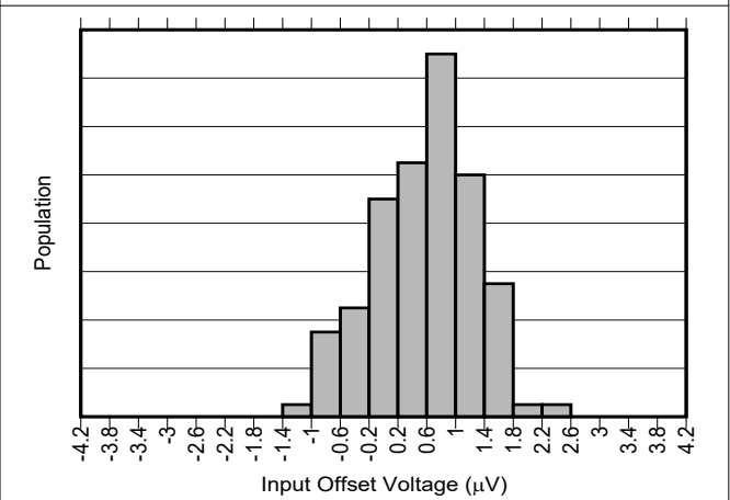
图 7-4. INA241A5-Q1 输入失调电压产生分布图
