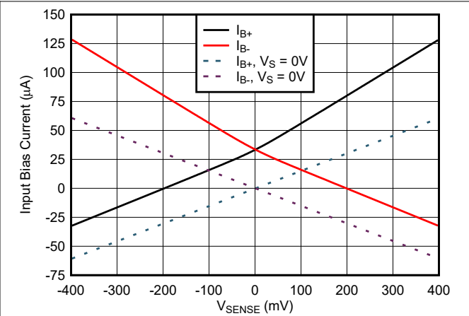
图 7-20. INA241x3-Q1 和 INA241x4-Q1 输入偏置电流与 V_{\text{SENSE}} 间的关系
