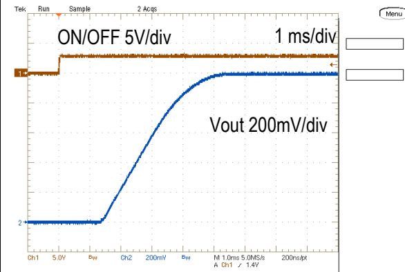
On/Off Enable Delay (Vin=12V, Vout=1.0V, Iout=4A, Cload=400uF)
