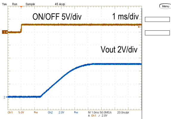
On/Off Enable Delay (Vin=12V, Vout=5.0V, Iout=4A, Cload=400uF)
