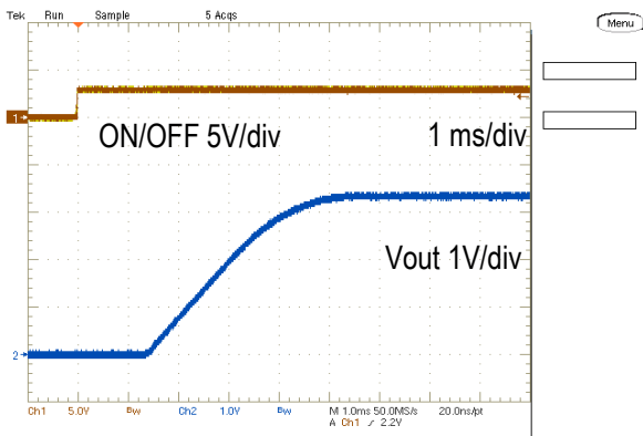
On/Off Enable Delay (Vin=12V, Vout=3.3V, Iout=4A, Cload=400uF)
