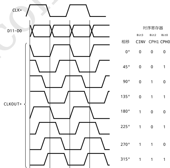
图 13: 相位偏移
