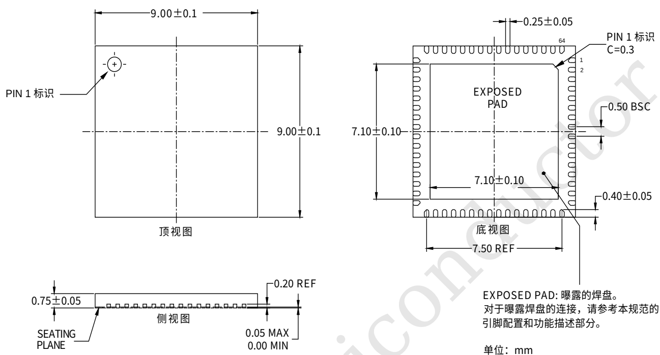
图 15: 封装信息
