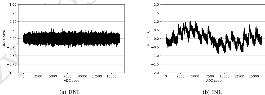
图 3: 线性特性
