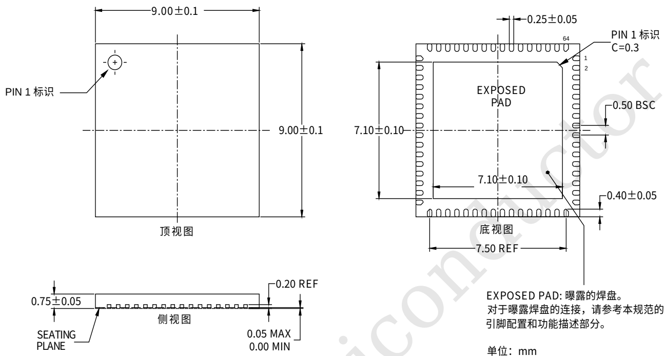
图 15: 封装信息
