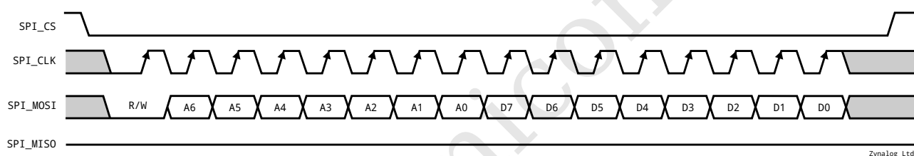
图 14: SPI 时序图
