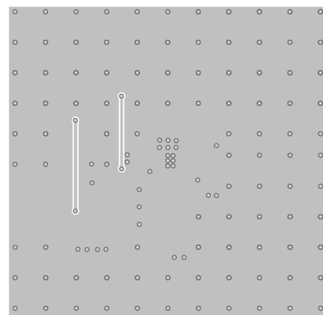
Bottom Layer
