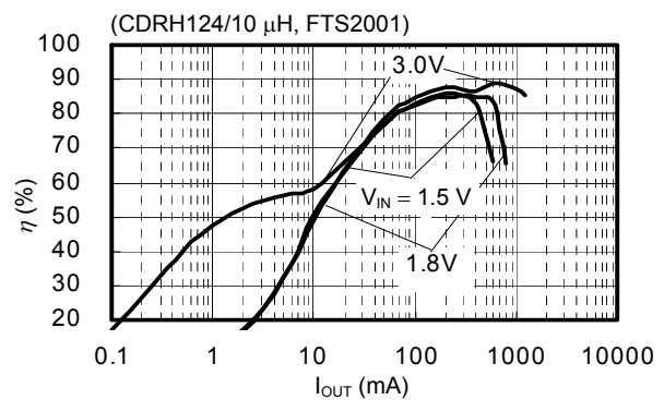
(8) S-8341A33AFT
