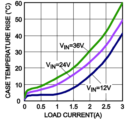
Thermal Rise
