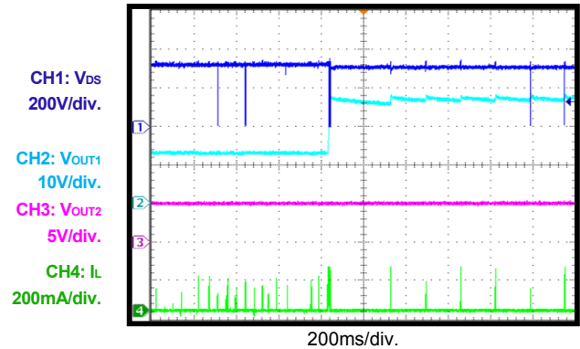
V_{OUT1} OVP No Load
