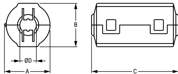
ESD-SR-S Type
