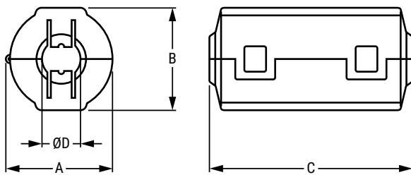
ESD-SR Type
