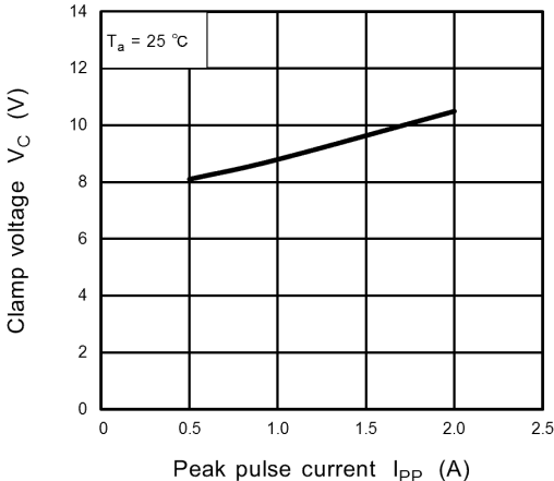
Fig. 6.2.1 V_C - I_{PP}
