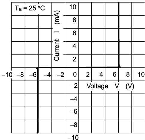
Fig. 9.1 I - V
