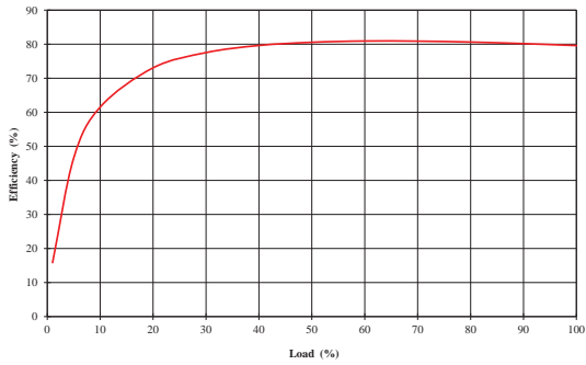
12V INPUT
