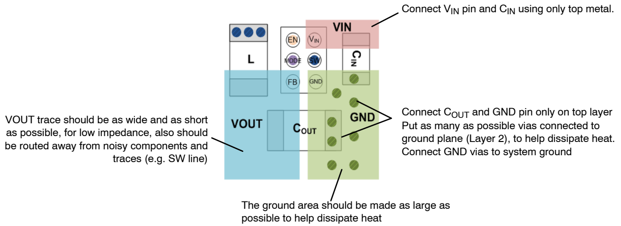
Figure 22. Top Layer
