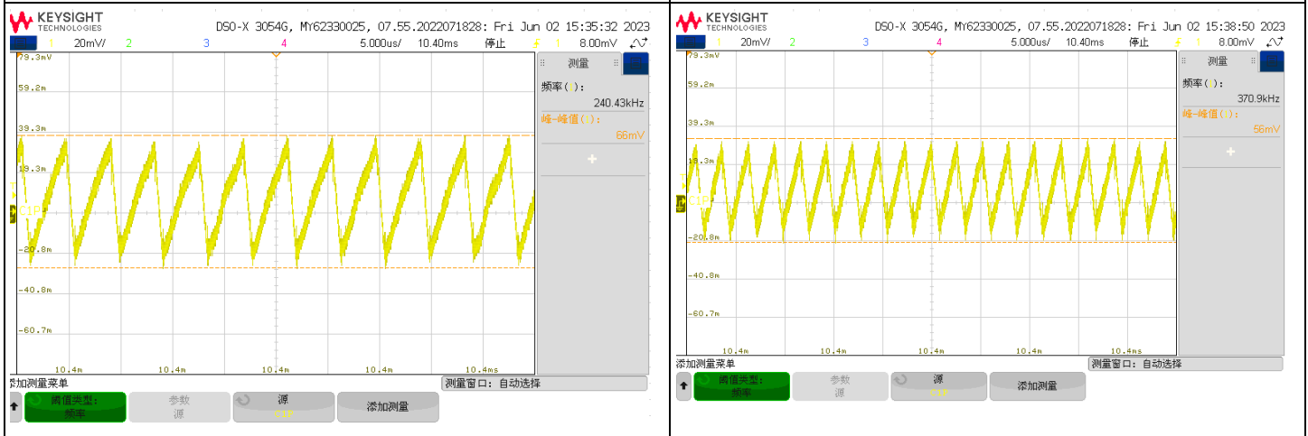
VINP=5V, VISO=5V, IISO=300mA, VISO 纹波电压峰峰值
