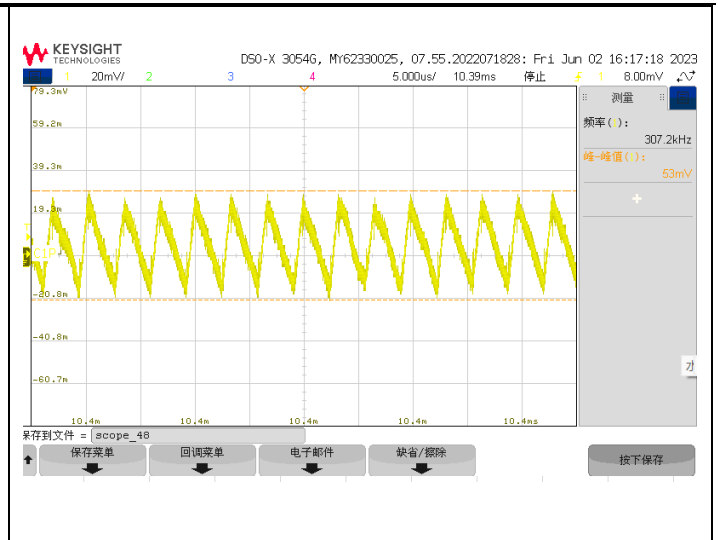
VINP=5V, VISO=3.7V, IISO=300mA, VISO 纹波电压峰峰值
