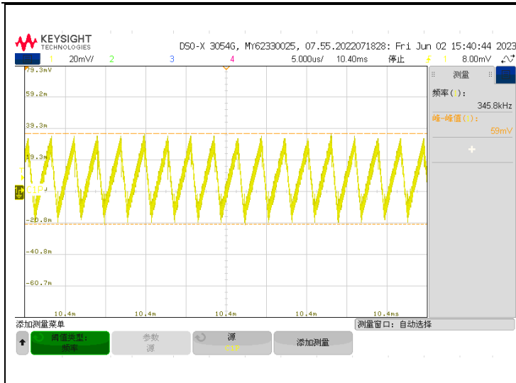
VINP=5V, VISO=5.4V, IISO=300mA, VISO 纹波电压峰峰值
