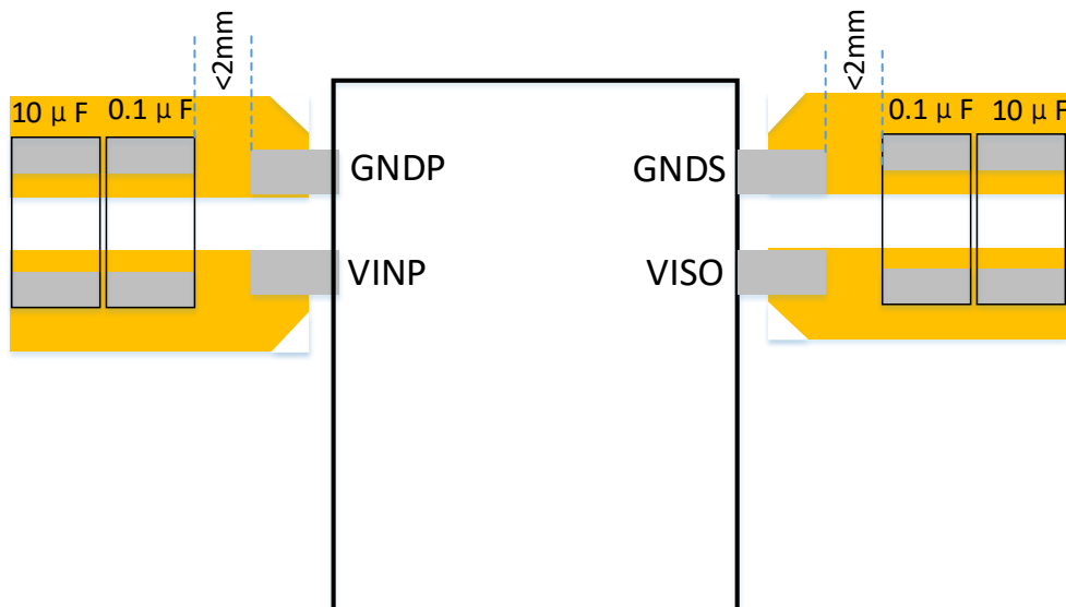
图 11-1 推荐电源部分 PCB 走线
